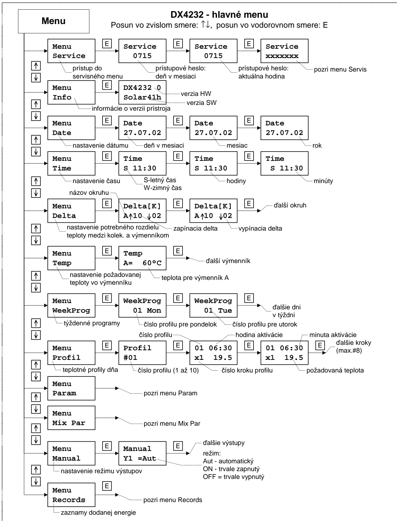
Obr.16 Menu regulátora DX4232 - menu pre servis je popísané na Obr.19
