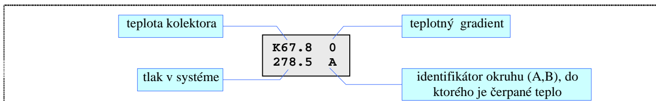
Obr.30 Zobrazenie tlaku v systéme
