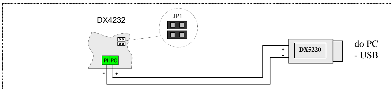
Obr.39 Pripojenie prístroja k PC s vnútorným napájaním (na PI-PO je naprázdno približne 14V, po pripojení prevodníka je na PI-PO 2,7V).
