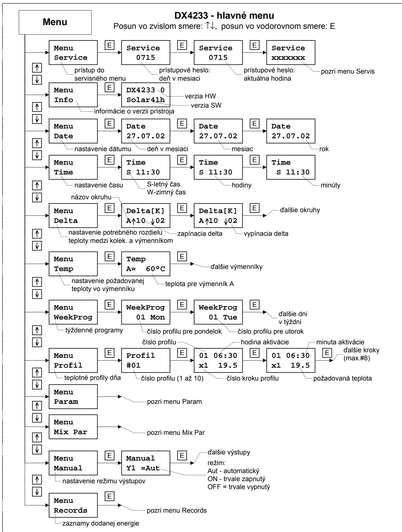
Obr.16 Menu regulátora DX4233 - menu pre servis je popísané na Obr.19
