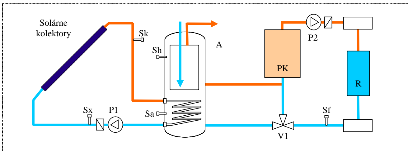
Obr.8 Príklad schémy regulovanej sústavy s diferenciálnym ohrevom: A - akumul. nádrž, PK - kotol, Sk, Sx, Sa, Sh, Sf - snímače teploty, V1 - prepínací ventil, P1, P2 - čerpadla, R - vykurovacie teleso
