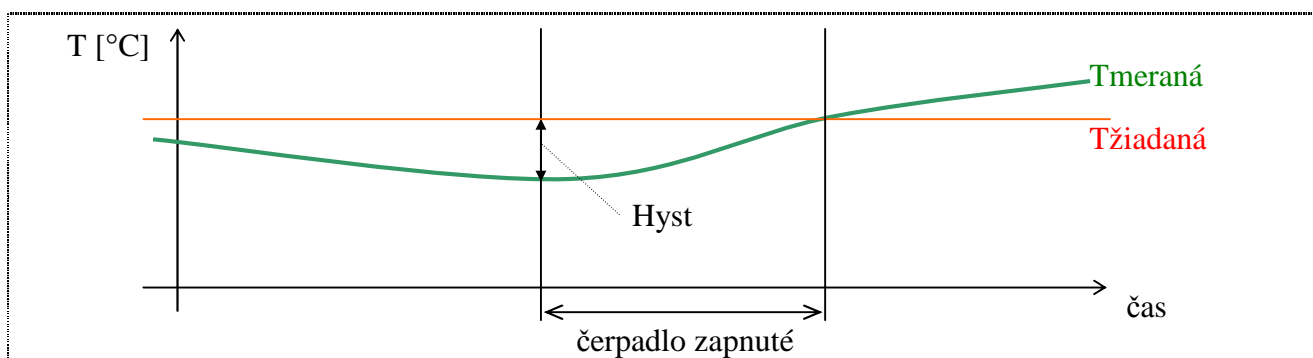
Obr.11 Princíp regulácie teploty objektu
