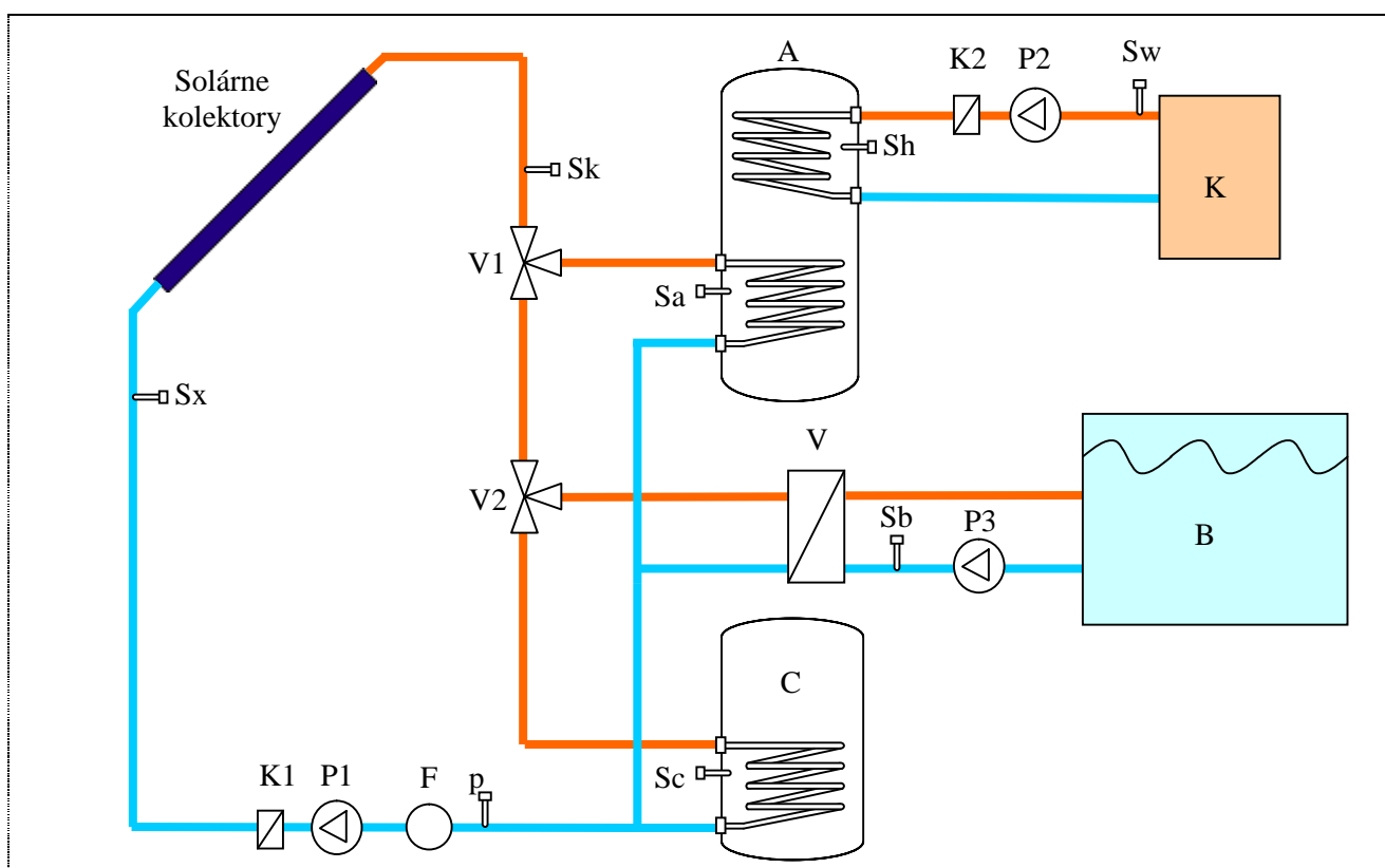
Obr.2 Hydraulická schéma regulovanej sústavy s prepínacími ventilmi: A - výmenník (bojler), V - doskový výmenník (pre bazén B), C - výmenník (akum. nádrž), Sk, Sa, Sb, Sc, Sx, Sh, Sw - snímače teploty, p - snímač tlaku, F - snímač prietoku, V1, V2 - prepínacie ventily, P1, P2, P3 - čerpadla, K - kotol (alebo krb), K1, K2 - spätné klapky
