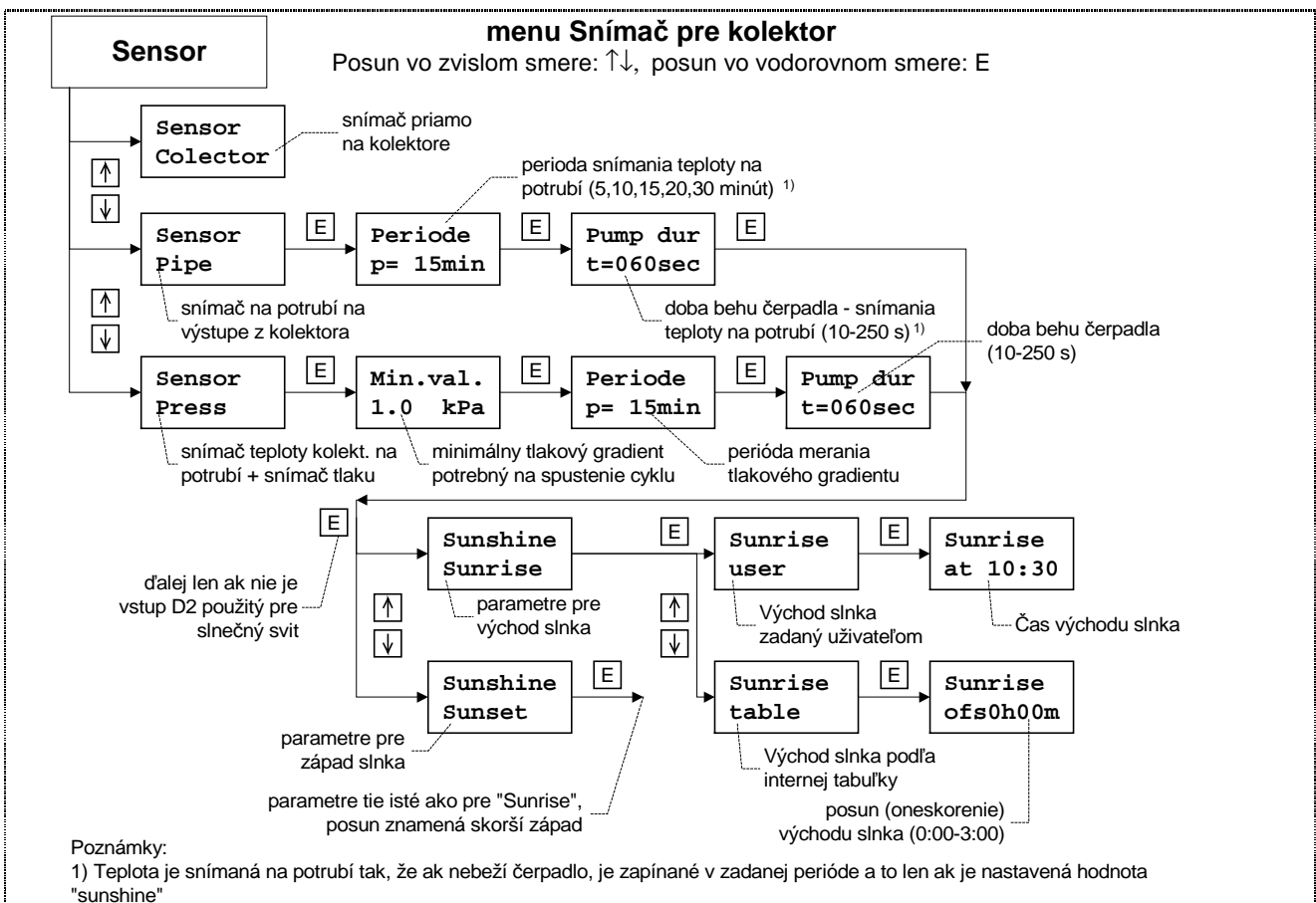
Obr.22 Menu "Sensor" - pre snímání teploty kolektora
