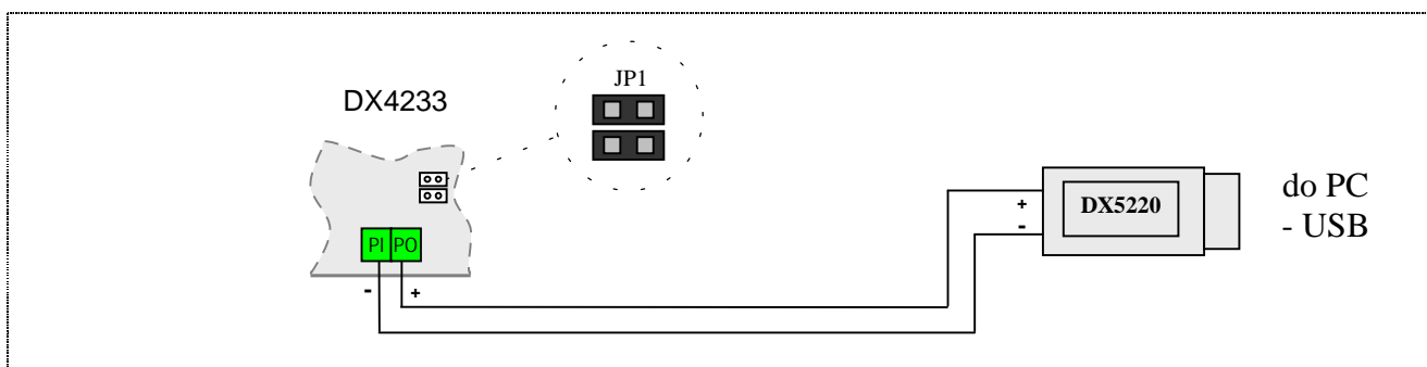
Obr.40 Pripojenie prístroja k PC s vnútorným napájaním (na PI-PO je naprázdno približne 14V, po pripojení prevodníka je na PI-PO 2,7V).
