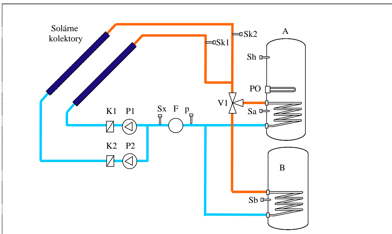
Obr.4 Hydraulická schéma regulovanej sústavy s dvoma kolektorovými poliemi: A, B - výmenníky, Sk1, Sk2, Sa, Sb, Sx, Sh - snímače teploty, p - snímač tlaku, F - snímač prietoku, PO - pomocný ohrev, V1 - prepínací ventil, P1,P2 - čerpadlá, K1,K2 - spätné klapky
