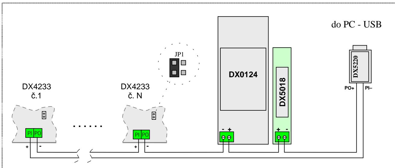
Obr.41 Pripojenie viacerých prístrojov k PC s vonkajším napájaním (na PI-PO je približne 2,1V). Keďže napájací zdroj DX0124 má max. 28 V (napätie je nastaviteľné), je možné pripojiť max. 10 prístrojov. V prípade potreby pripojenia viacej ako 10 prístrojov je potrebné použiť napájací zdroj z väčším napätím ( n * 2,1 + 5 ) alebo zapojiť do série dva zdroje DX0124.
