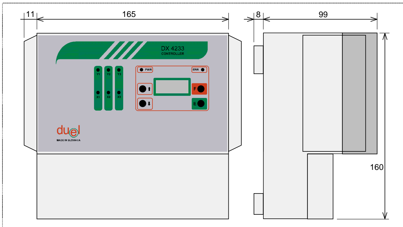
Obr.36 Rozmery prístroja DX4233
