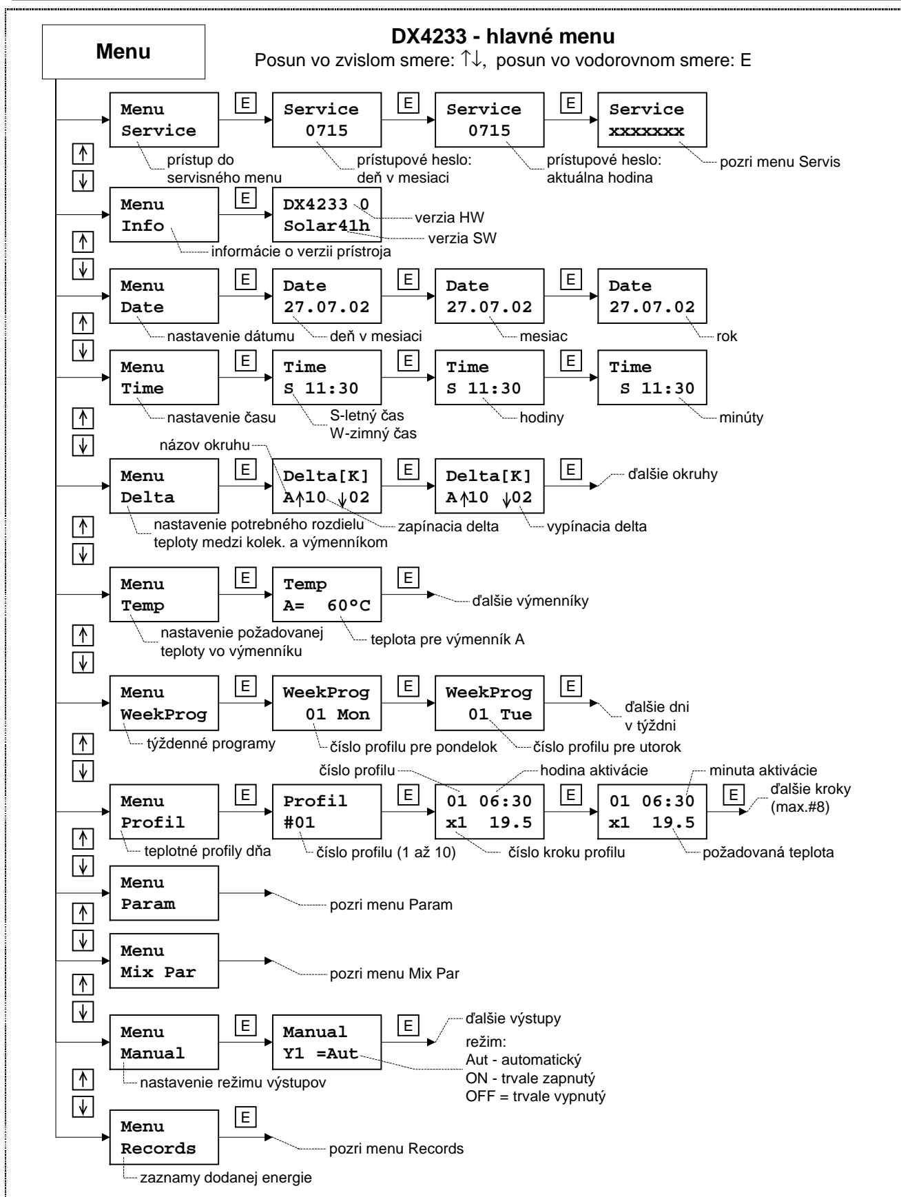
Obr.17 Menu regulátora DX4233 - menu pre servis je popísané na Obr.20
