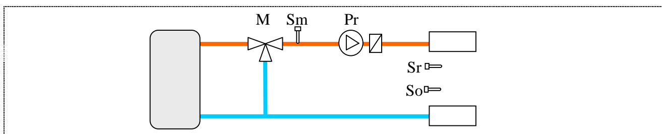
Obr.11 Schéma ekvitermickej regulácie
