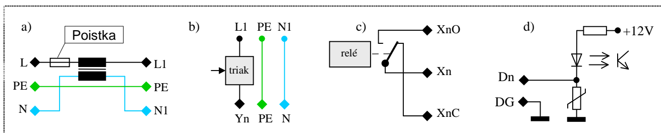
Obr.38 Zapojenia prístroja DX4233: a) prepojenie vstupného napätia b) výstupy Y1-Y3, c) výstupy X1-X3, d) digit. vstupy D1 a D2
