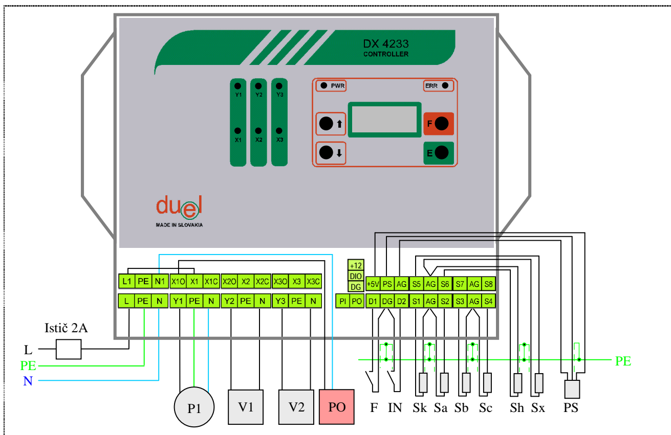
Obr.39 Príklad zapojenia regulátora DX4233 (svorkovnice sú pod krytom) pre sústavu s prepínacími ventilmi: Sk - snímač teploty kolektora, Sa, Sb, Sc - snímače teplôt výmenníkov, Sx - snímač teploty spätného toku, Sh - snímač teploty pomocného ohrevu, PS - snímač tlaku, F - impulzný prietokomer, IN - prepínanie leto/zima, P1 - čerpadlo, V1, V2 - prepínacie ventily, PO - stýkač, ktorý spína pomocný ohrev
