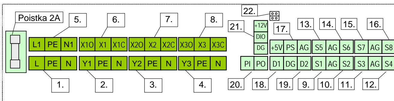
Obr.37 Zapojenie svorkovnice regulátora DX4233
