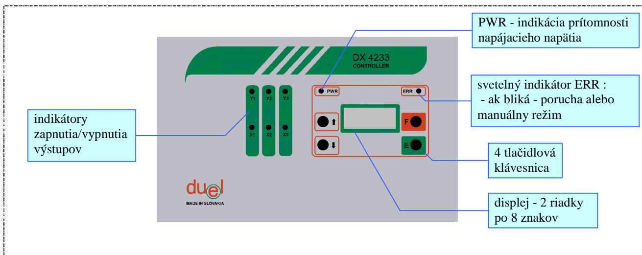
Obr.14 Predný panel regulátora DX4233
