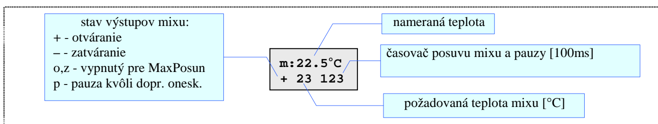
Obr.34 Zobrazenie stavu mixu
