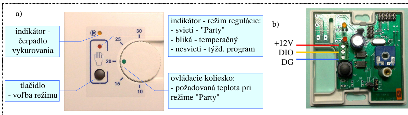
Obr.43 Priestorový snímač teploty DX1081: a) pohľad spredu, b) pohľad dovnútra a pripojenie k DX4233
