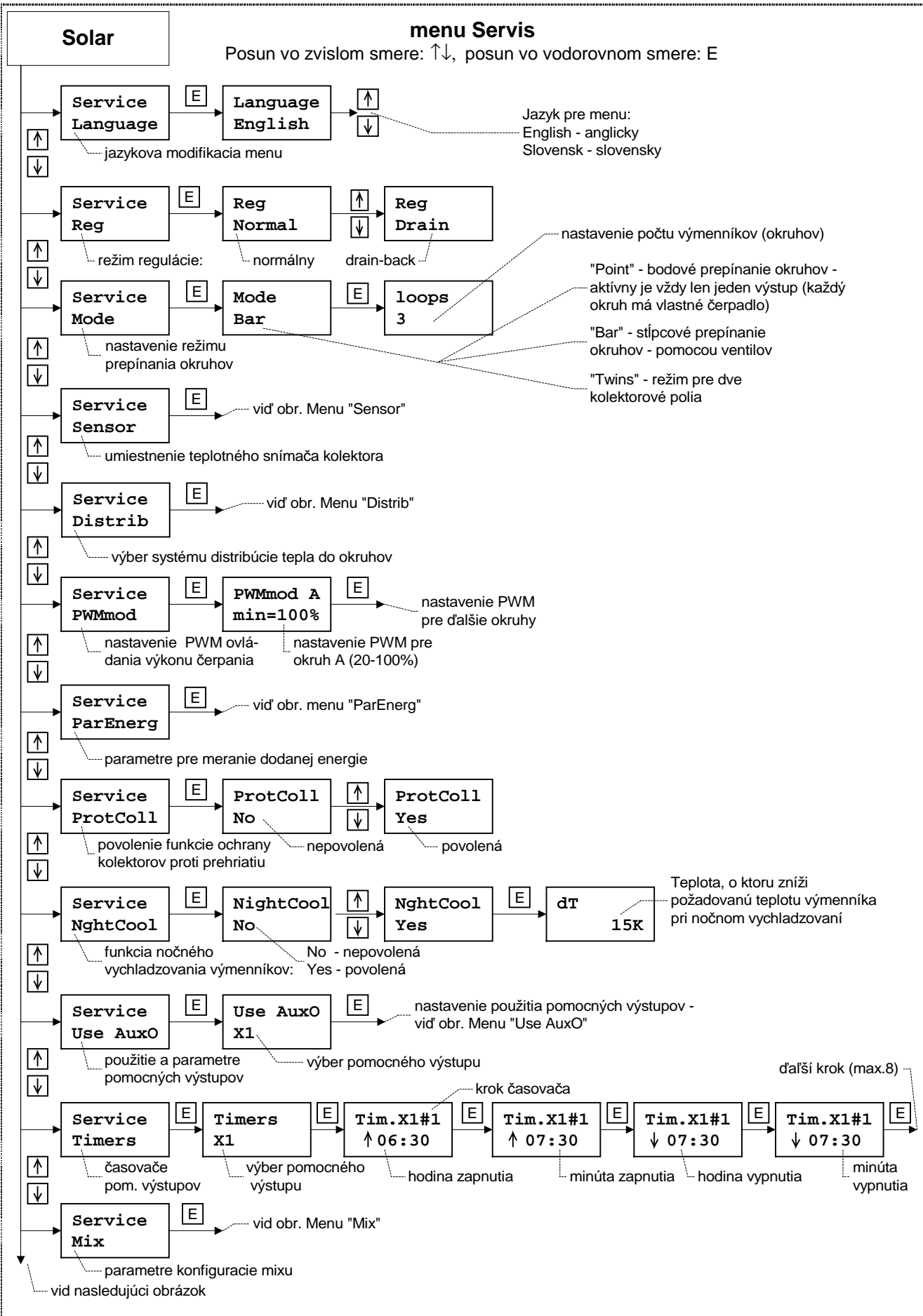
Obr.20 Menu Servis - 1.časť
