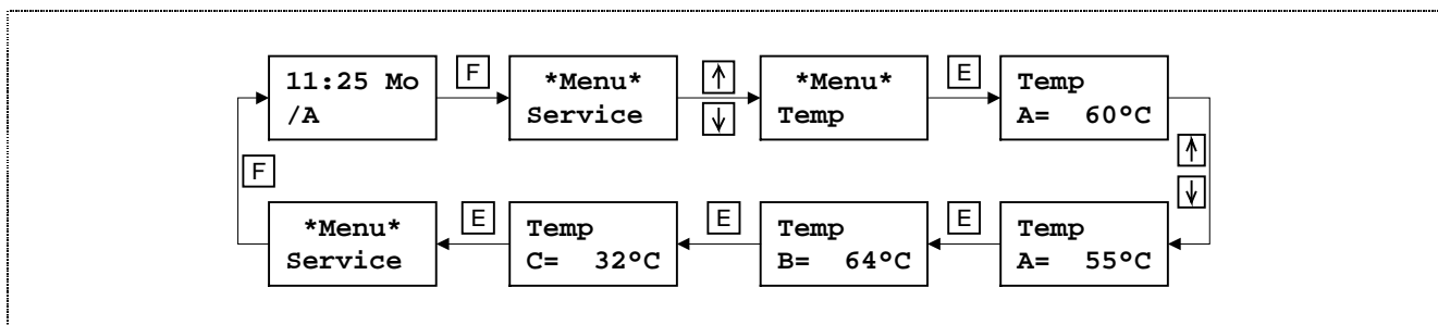
Obr.16 Príklad nastavenia požadovanej teploty
