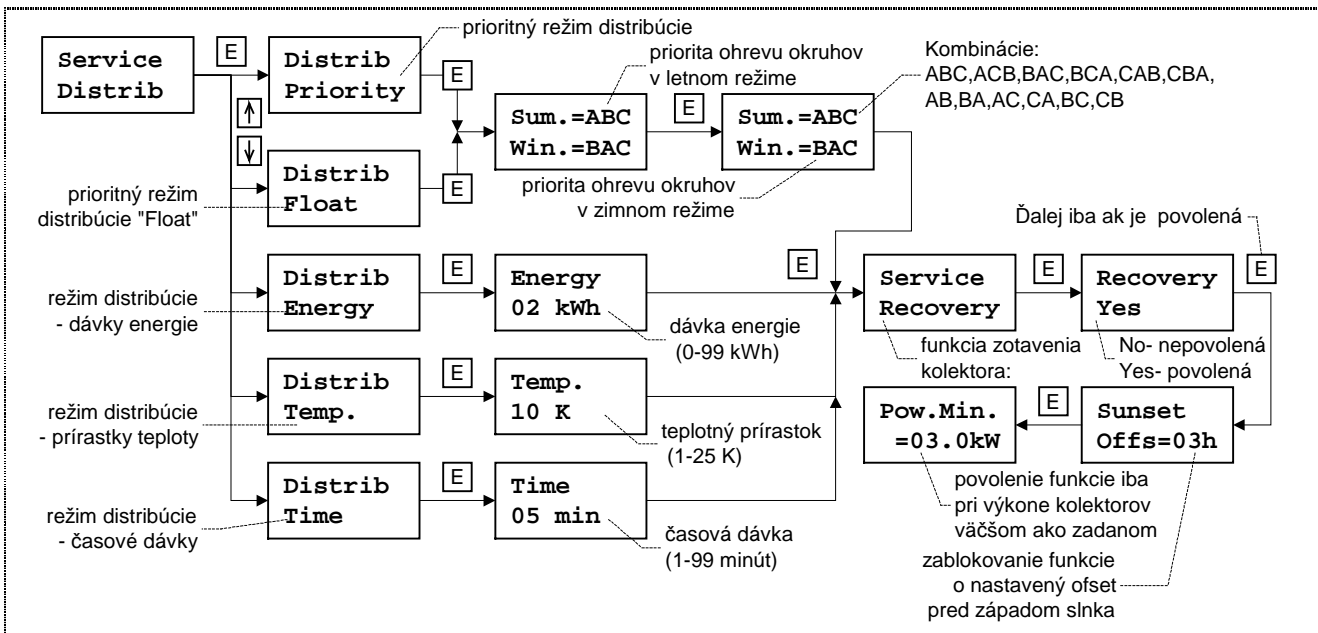
Obr.23 Menu "Distrib" - distribučné režimy
