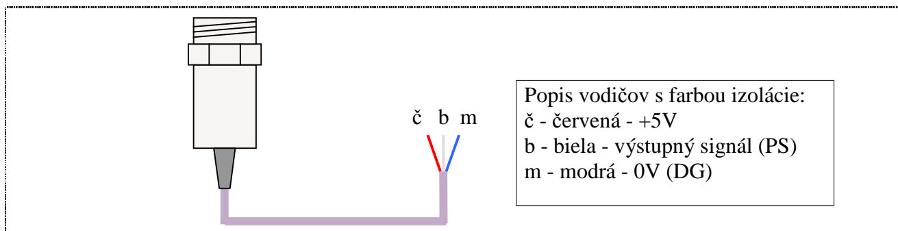
Obr.42 Snímač tlaku DX5500
