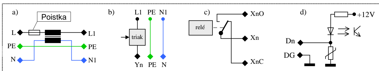
Obr.38 Zapojenia prístroja DX4232: a) prepojenie vstupného napätia b) výstupy Y1-Y2, c) výstupy X1-X2, d) digitálne vstupy D1 a D2
