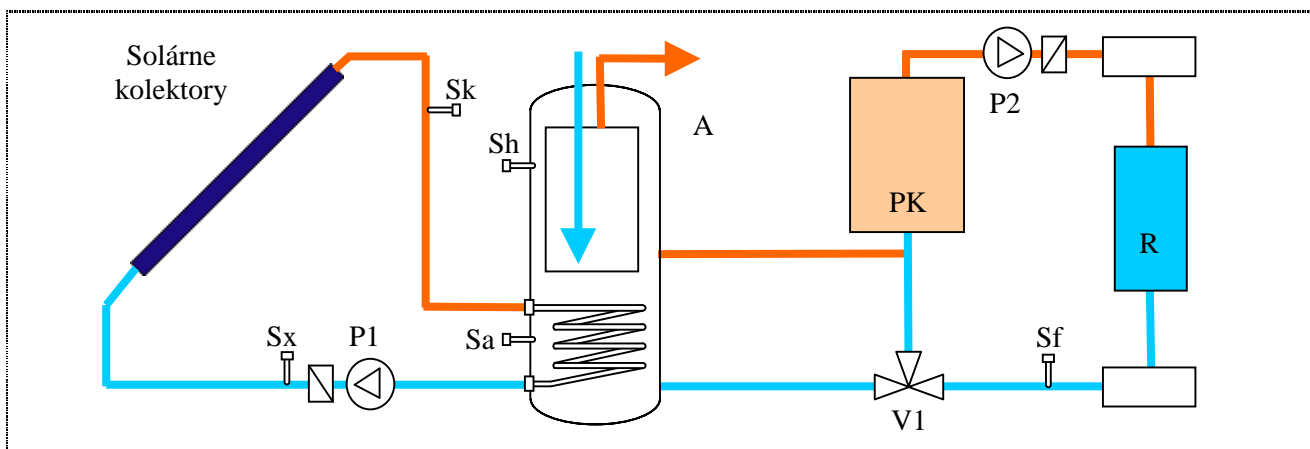
Obr.8 Príklad schémy regulovanej sústavy s diferenciálnym ohrevom: A - akumul. nádrž, PK - kotol, Sk, Sx, Sa, Sh, Sf - snímače teploty, V1 - prepínací ventil, P1, P2 - čerpadla, R - vykurovacie telesa
