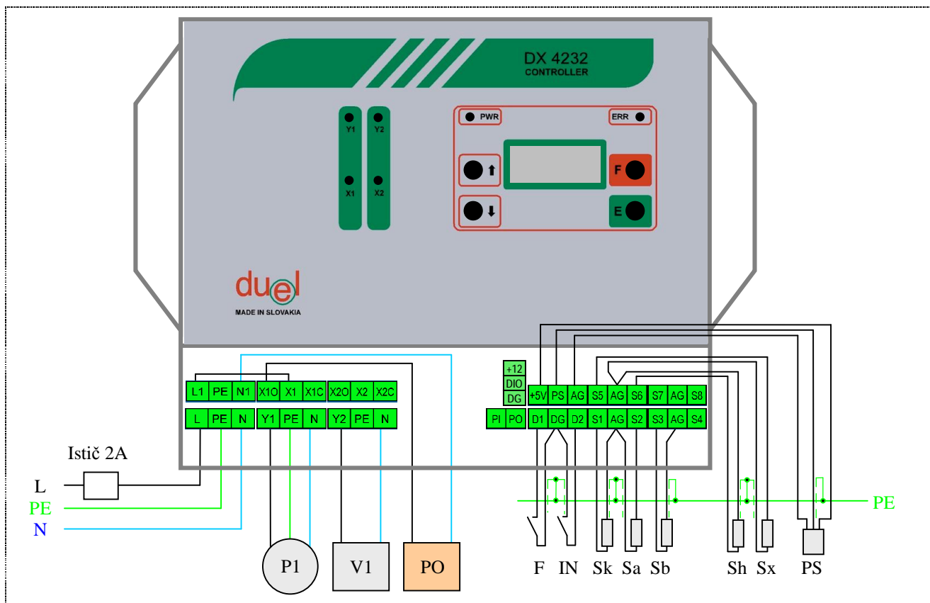
Obr.39 Príklad zapojenia regulátora DX4232 (svorkovnice sú pod krytom) pre sústavu s prepínacím ventilom: Sk - snímač teploty kolektora, Sa, Sb - snímače teplôt výmenníkov, Sx - snímač teploty spätného toku, Sh - snímač teploty pomocného ohrevu, PS - snímač tlaku, P1 - čerpadlo, V1 - prepínací ventil, F - impulzný prietokomer, IN - prepínanie leto/zima, PO - stýkač, ktorý spína pomocný ohrev
