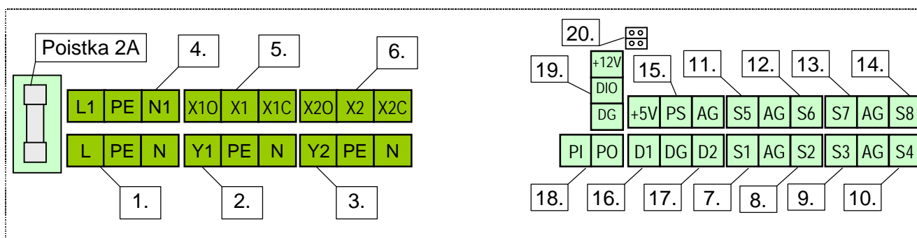
Obr.37 Zapojenie svorkovnice regulátora DX4232
