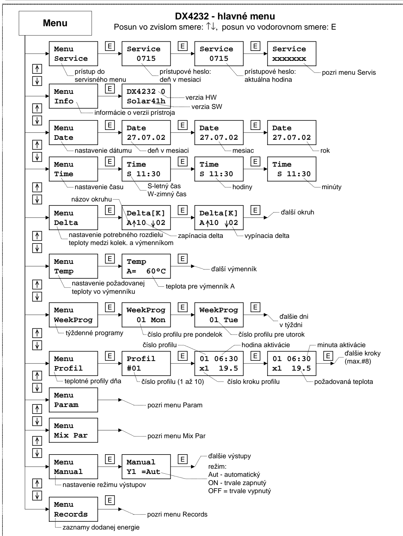
Obr.17 Menu regulátora DX4232 - menu pre servis je popísané na Obr.20
