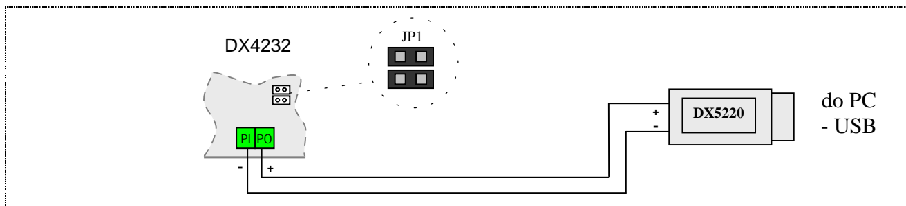
Obr.40 Pripojenie prístroja k PC s vnútorným napájaním (na PI-PO je naprázdno približne 14V, po pripojení prevodníka je na PI-PO 2,7V).
