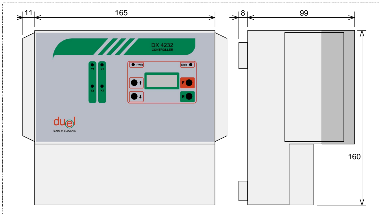
Obr.36 Rozmery prístroja DX4232
