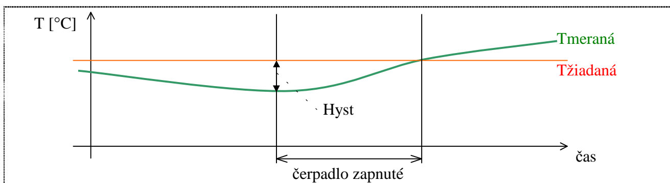
Obr.12 Princíp regulácie teploty objektu
