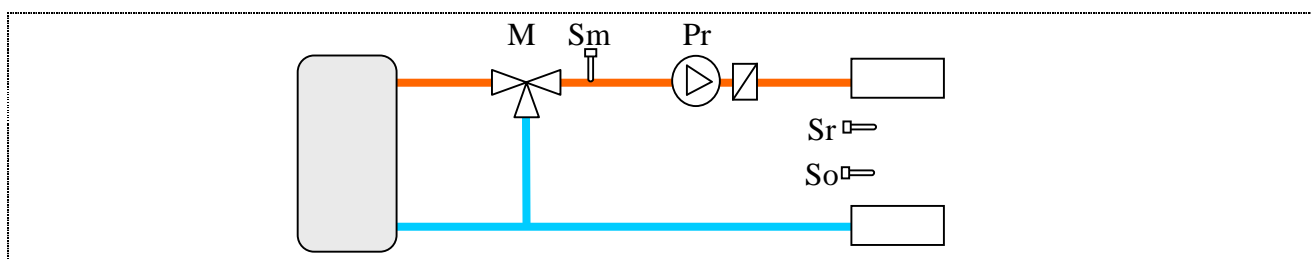
Obr.11 Schéma ekvitermickej regulácie
