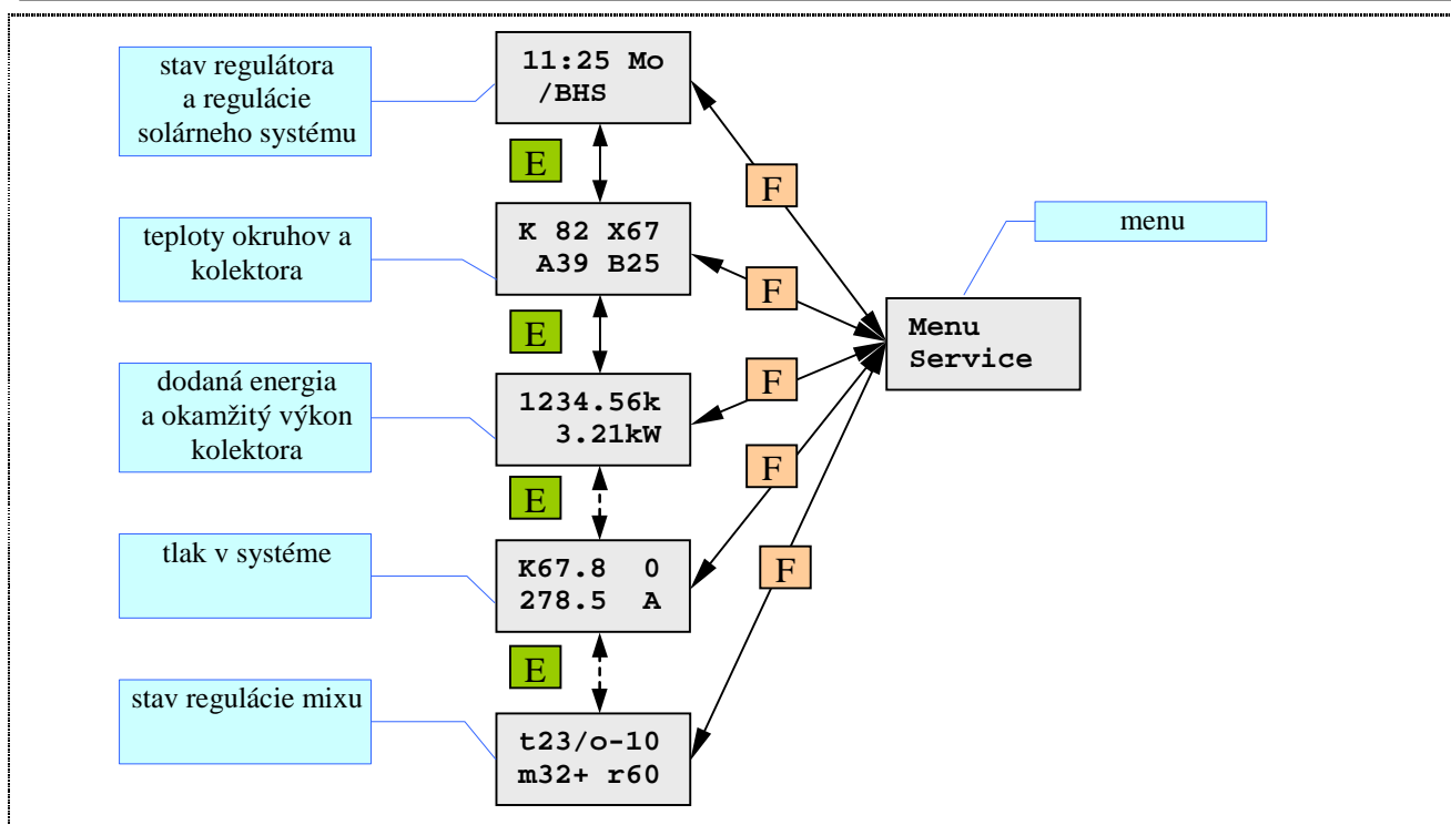
Obr.15 Prepínanie medzi zobrazovaniami stavu regulácie a menu
