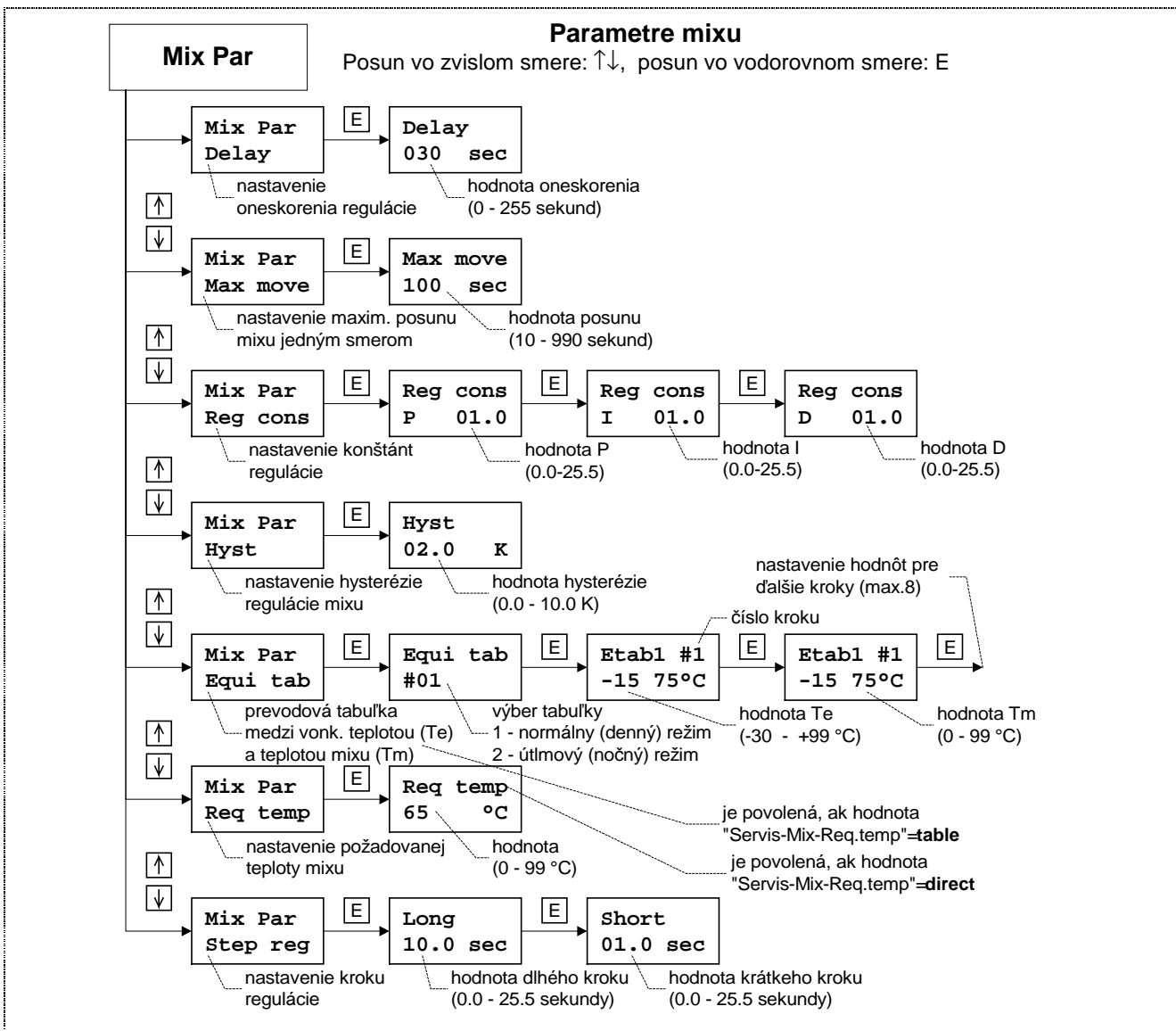
Obr.19 Menu "Mix Par" - parametre pre Mix
