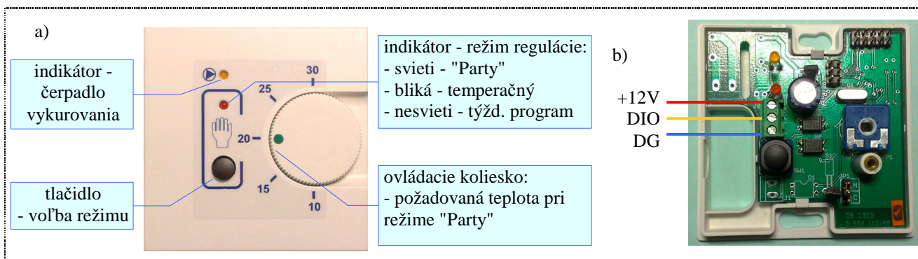
Obr.43 Priestorový snímač teploty DX1081: a) pohľad spredu, b) pohľad dovnútra a pripojenie k DX4232
